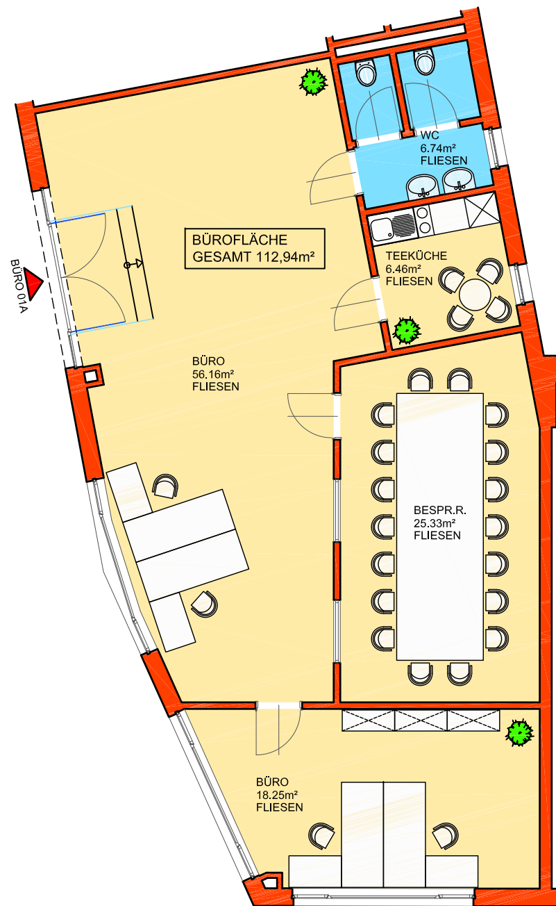
ERDGESCHOSS BÜRO 01A - 1:100
